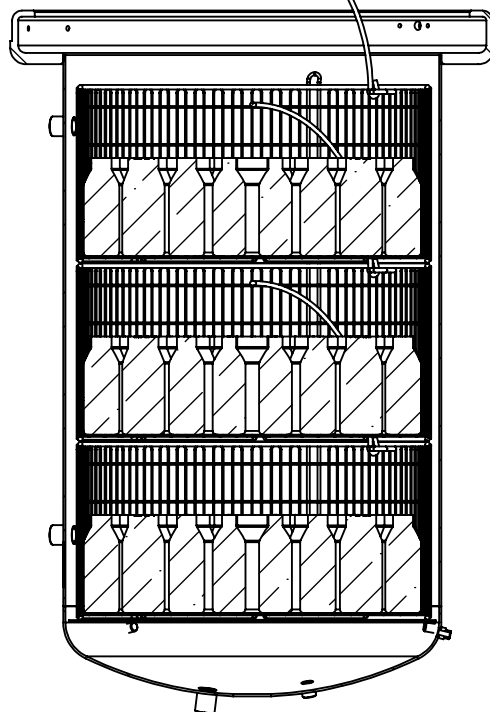
SECTION A-A
